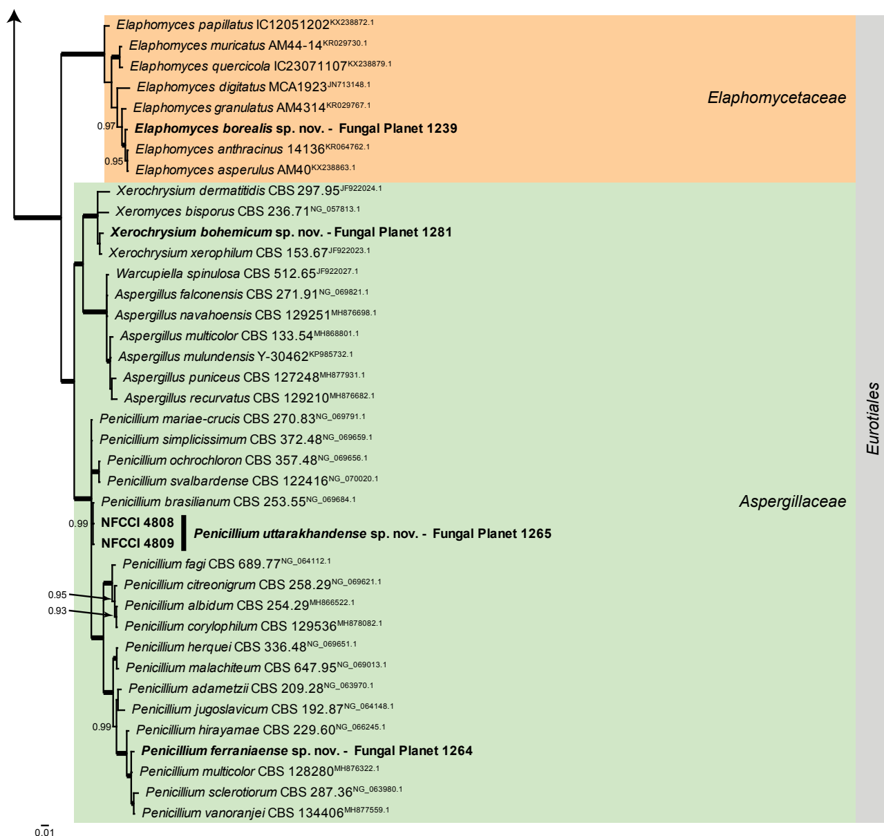
Overview Eurotiomycetes phylogeny – part 2
